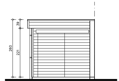
ZIJGEVEL RECHTS
