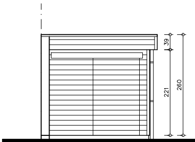
ZIJGEVEL LINKS
