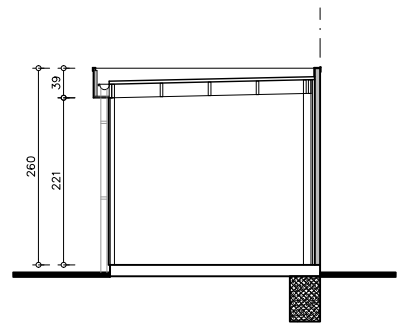
DOORSNEDE
