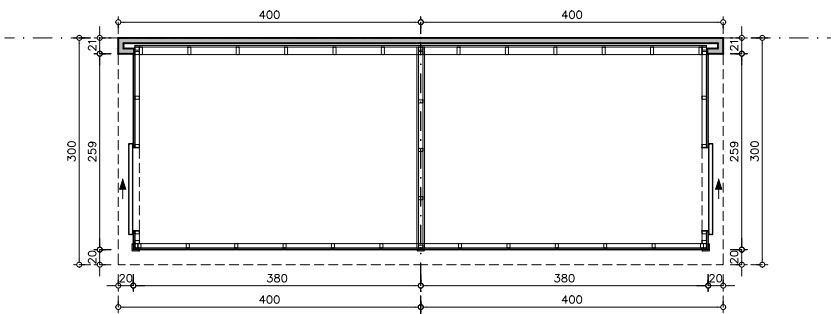
GRONDPLAN
