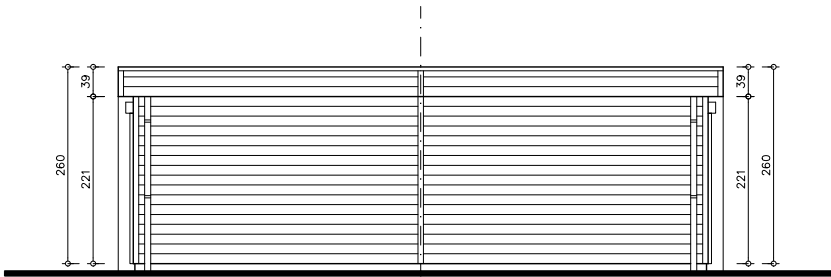
VOORGEVEL
